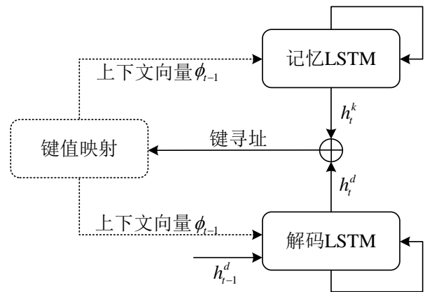
图 26 键寻址过程示意图
