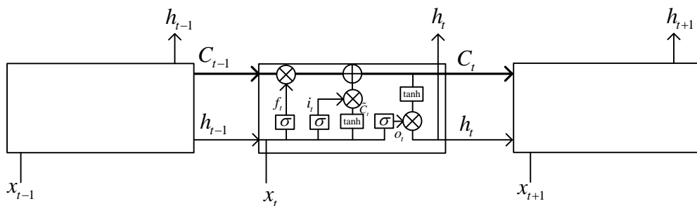
图 2 长短期记忆神经网络结构示意图
