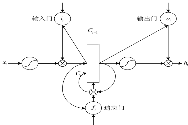
图 16 LSTMN 结构示意图
