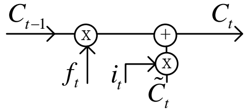
图5 单元状态更新示意图
