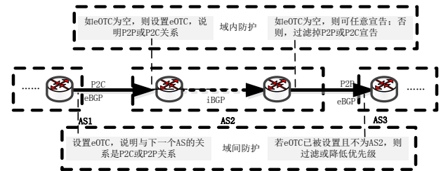
图 4 eOTC 路由泄露防护机制原理图
