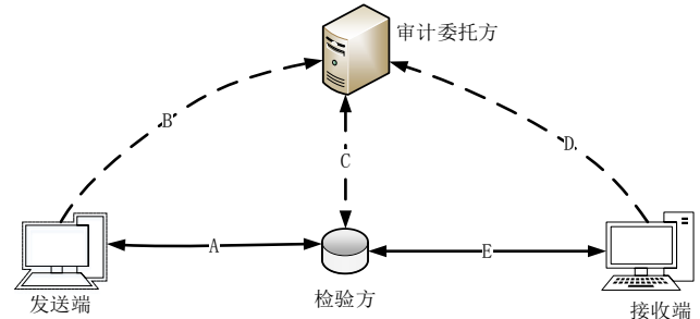
图 2 APIP 传输示意图
