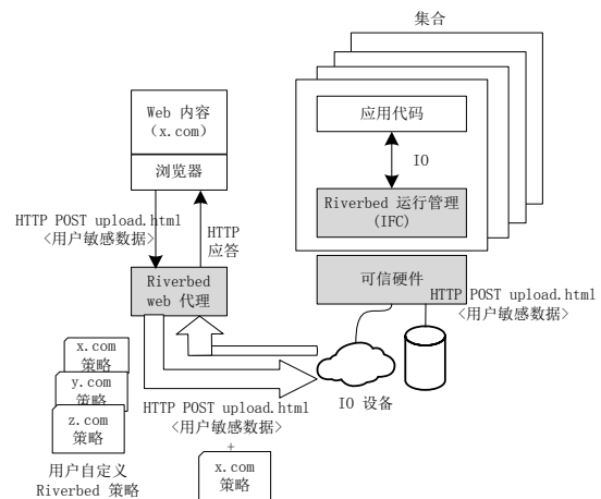
图5 Riverbed架构
