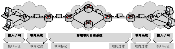
图 1 SAVA 架构图
