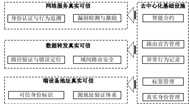
图 7 真实可信新一代互联网体系结构
