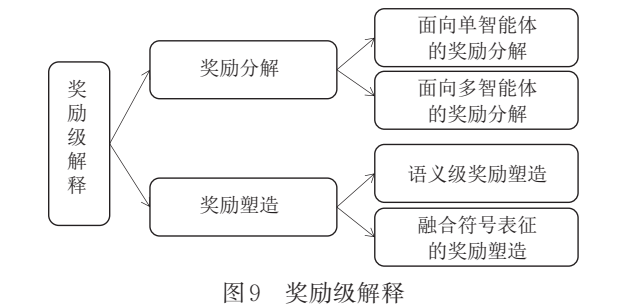
图9 奖励级解释
