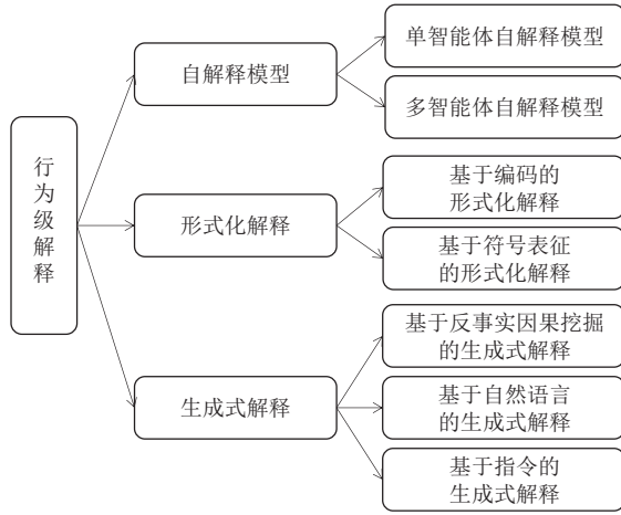
图2 行为级解释
