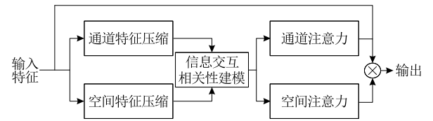
图 5 CBAM 与跨空间-通道注意力流程示意图
