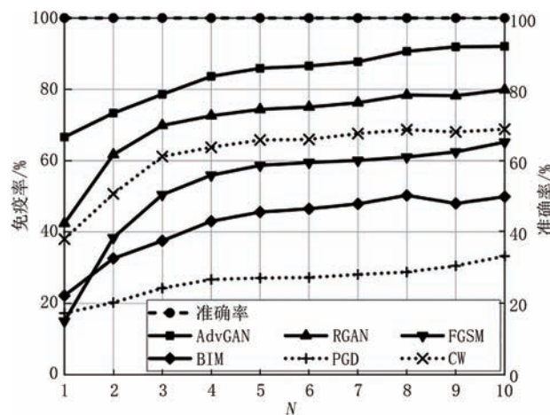
图4 在MNIST上,MID在不同的 N 值下针对AdvGAN制作的免疫样本的分类准确率(%)和免疫率(%),以及将免疫样本迁移至其他5种对抗攻击的免疫率(%)
