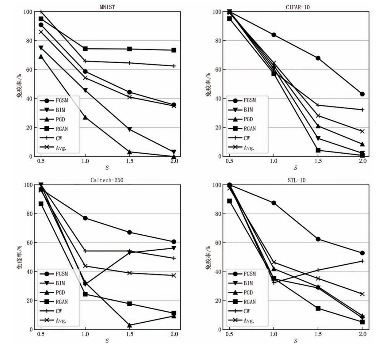
图 6 在 MNIST、CIFAR-10、STL-10 和 Caltech-256 上,使用 MID 针对 AdvGAN 制作的免疫样本并将免疫样本迁移至其他多种不同扰动强度的对抗攻击的免疫率(%) (Avg. 表示平均免疫率值)
