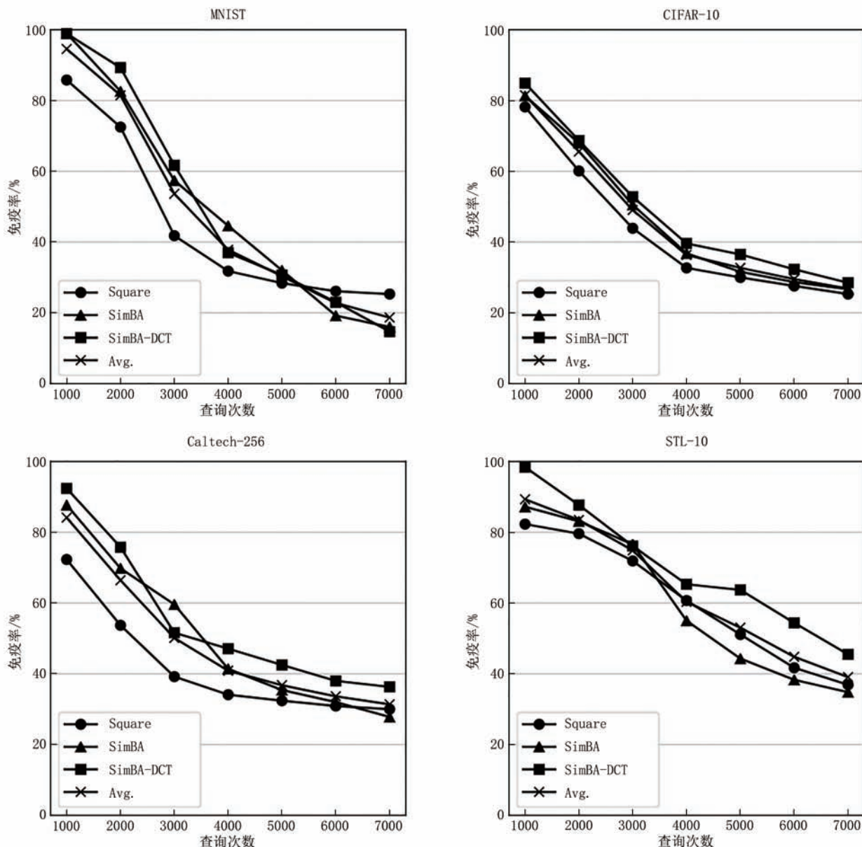
图7 在MNIST、CIFAR-10、STL-10和Caltech-256上,使用MID针对AdvGAN制作的免疫样本并将免疫样本迁移至其他多种不同查询次数的黑盒攻击的免疫率(%)(Avg.表示平均免疫率值)
