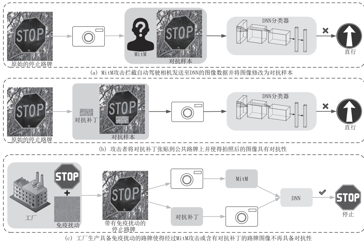
图1 对抗攻击和免疫防御的示意图
