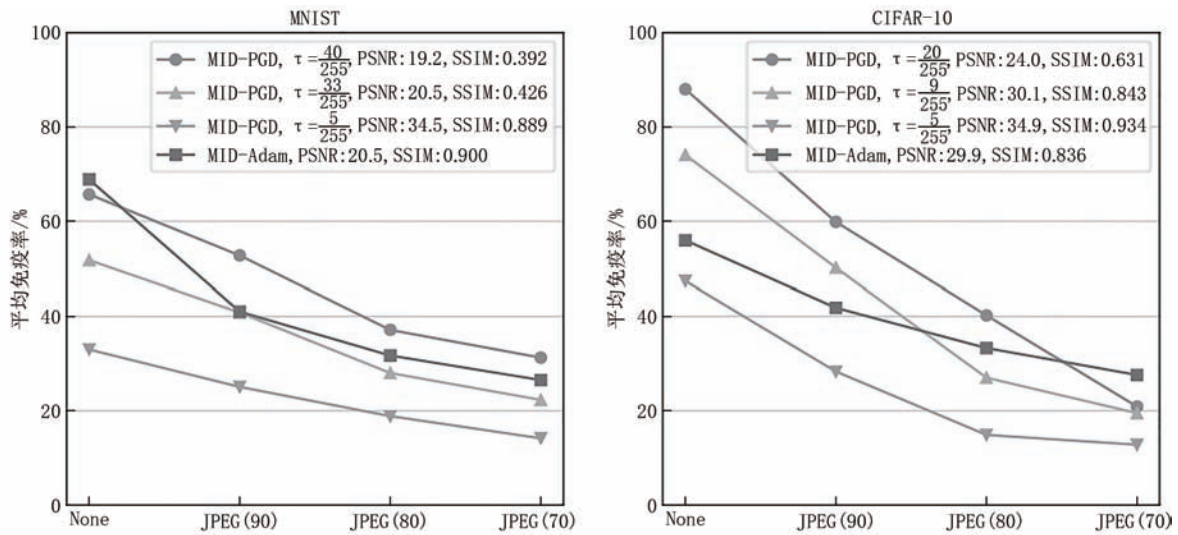
图9 MID-PGD和MID-Adam对不同质量因子的JPEG压缩的鲁棒性
