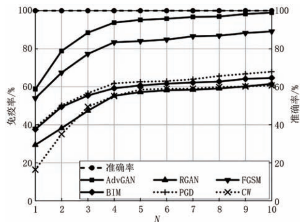
图3 在CIFAR-10上,MID在不同的 N 值下针对AdvGAN制作的免疫样本的分类准确率(%)和免疫率(%),以及将免疫样本迁移至其他5种对抗攻击的免疫率(%)
