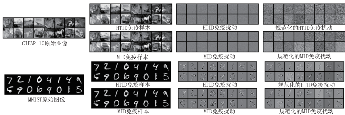
图 10 HTID 和 MID 在 CIFAR-10 和 MNIST 上制作的免疫样本
