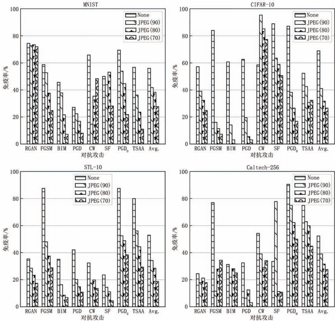
图8 在 MNIST、CIFAR-10、STL-10 和 Caltech-256 上, 使用 MID 针对 AdvGAN 制作的免疫样本并经过不同质量因子的 JPEG 压缩后的免疫率(%) (Avg. 表示平均免疫率值)
