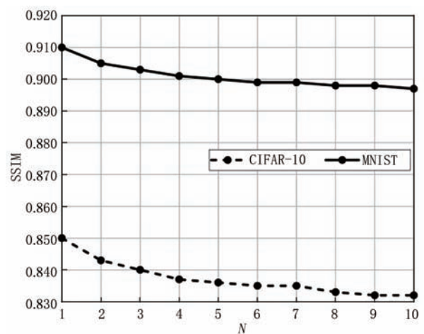
图5 在CIFAR-10和MNIST上,MID在不同的 N 值下针对AdvGAN制作的免疫样本的SSIM
