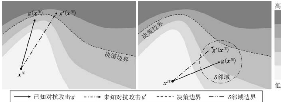
图2 HTID和MID制作的免疫样本防御对抗攻击的示意图(左图为HTID的示意图,右图为MID的示意图. x^{IE} 表示免疫样本, g(x^{IE}) 表示已知的对抗样本, g'(x^{IE}) 表示潜在的对抗样本. 图中颜色越深表示分类损失越大)
