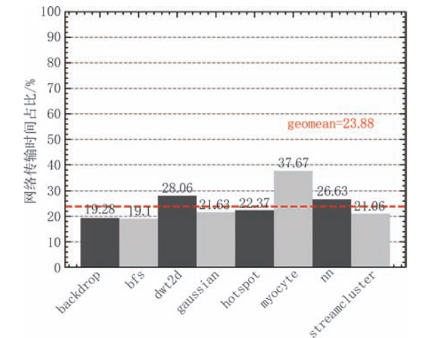
图8 云边协同下 gEdge 网络开销分析
