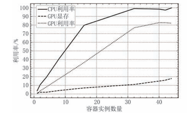
图14 容器密度实验
