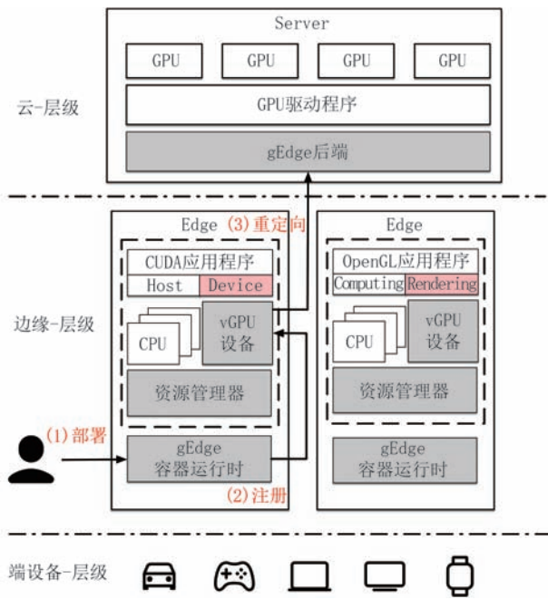
图3 gEdge架构图
