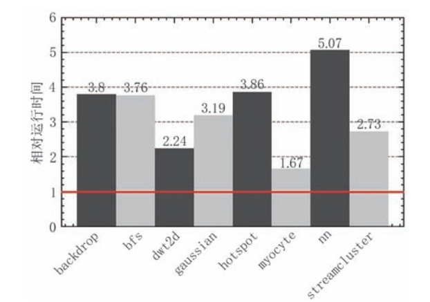
图7 云边协同下 gEdge 性能测试
