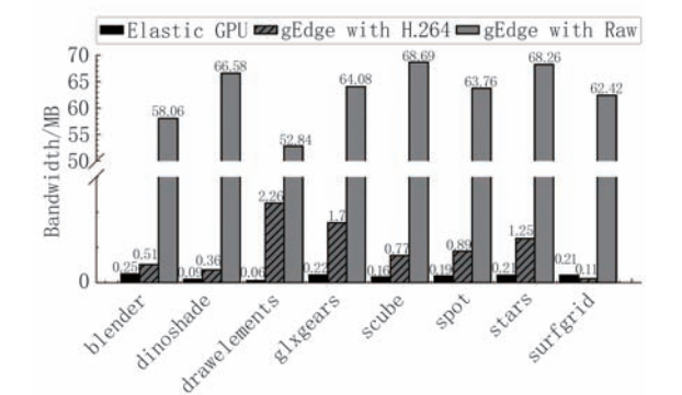
图13 带宽使用情况
